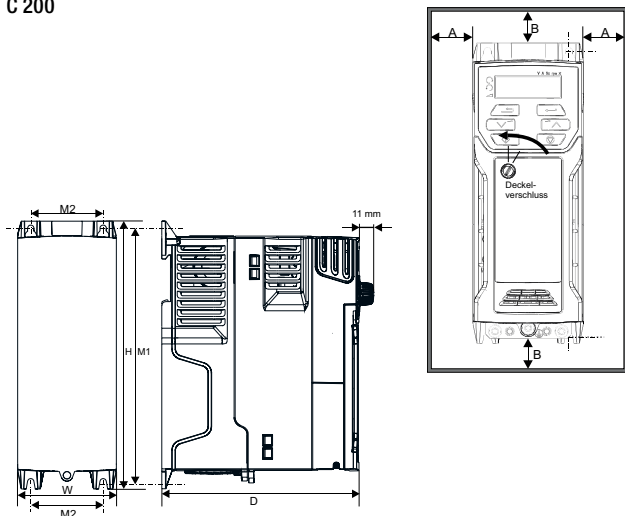
Medidas para instalación en mm C 200
